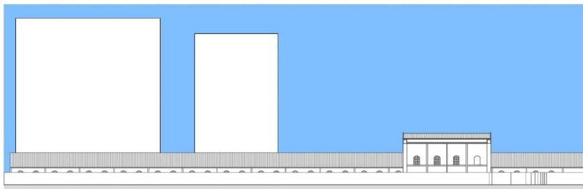
5 ELEVACÃO SUDESTE - Rua Vicente da Costa Braga (atual) ESCALA: gráfica
