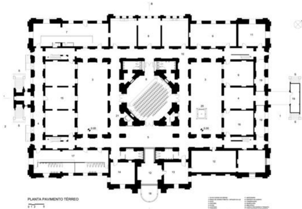
Figura 9 – Planta da Pinacoteca
