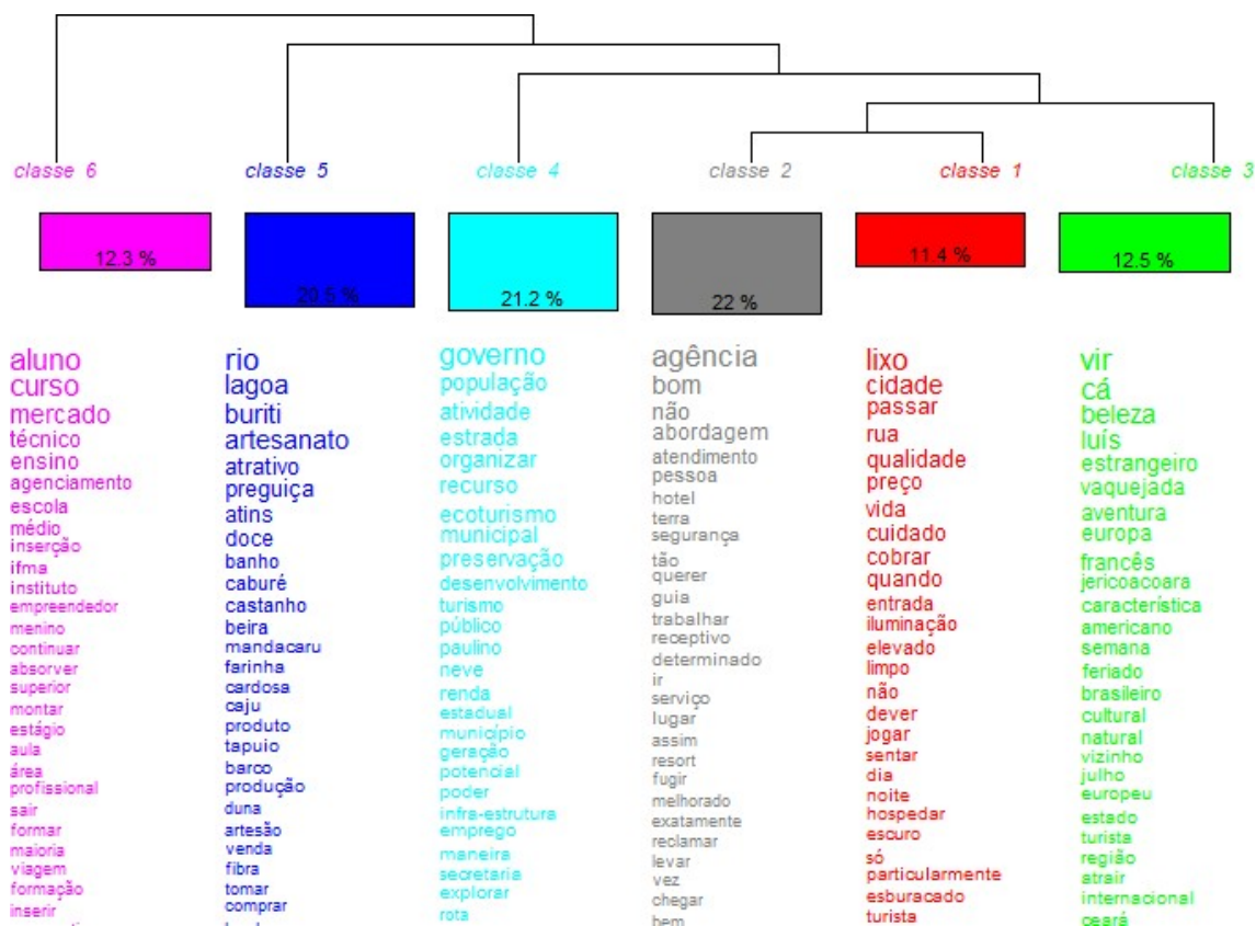
Figura 2. Dendograma
